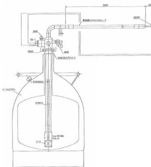
機器接続図(シーベル 30使用時)
