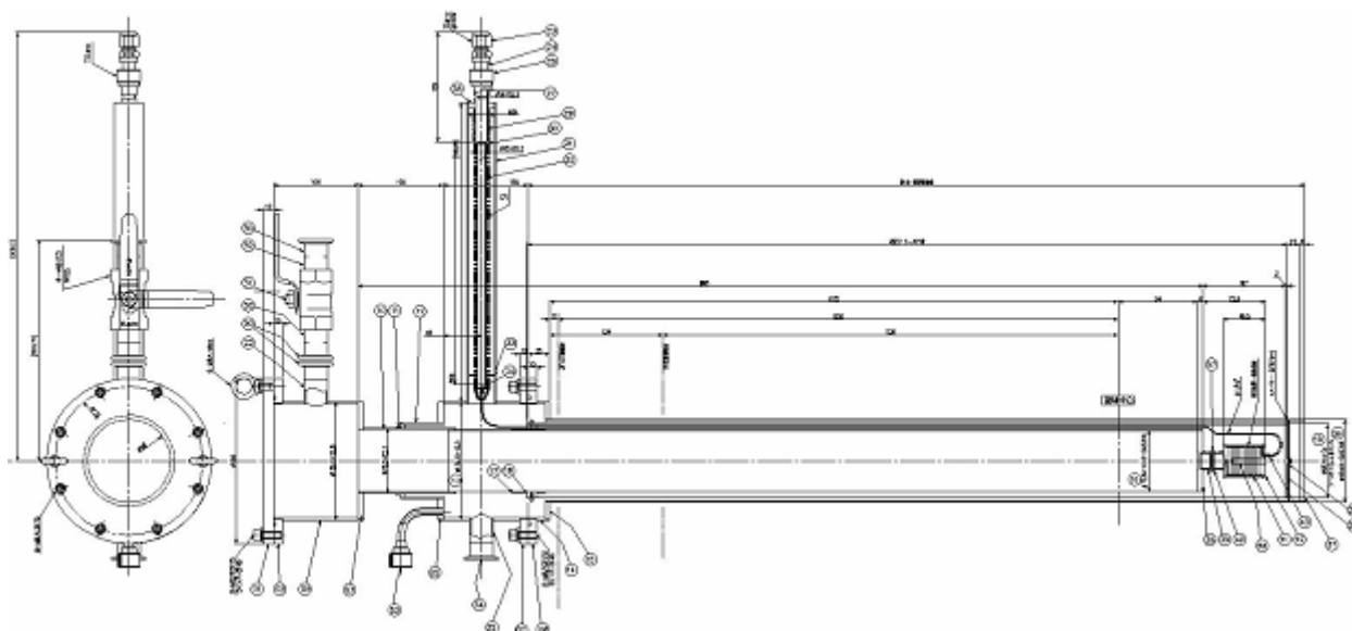
<本体外観図>
